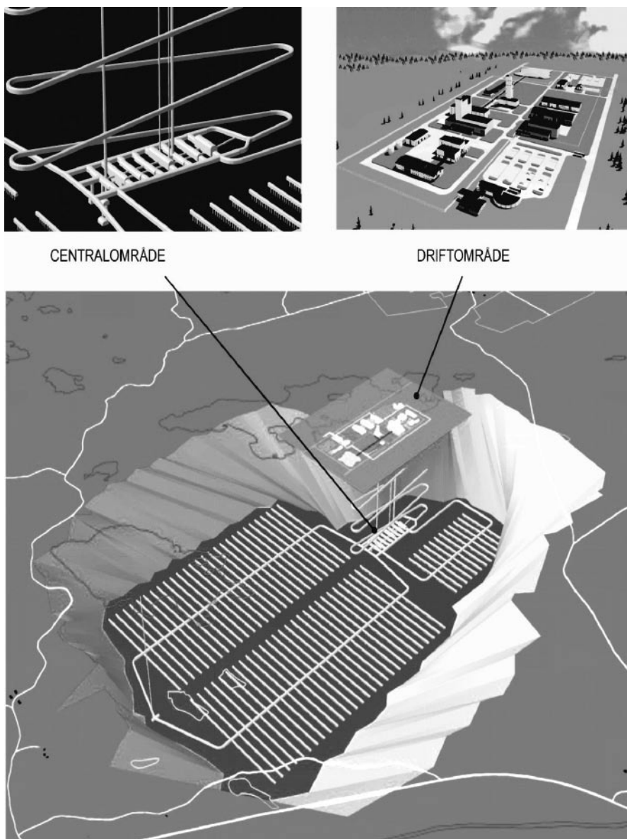
Figur 3-8. Slutförvaret – översikt.
