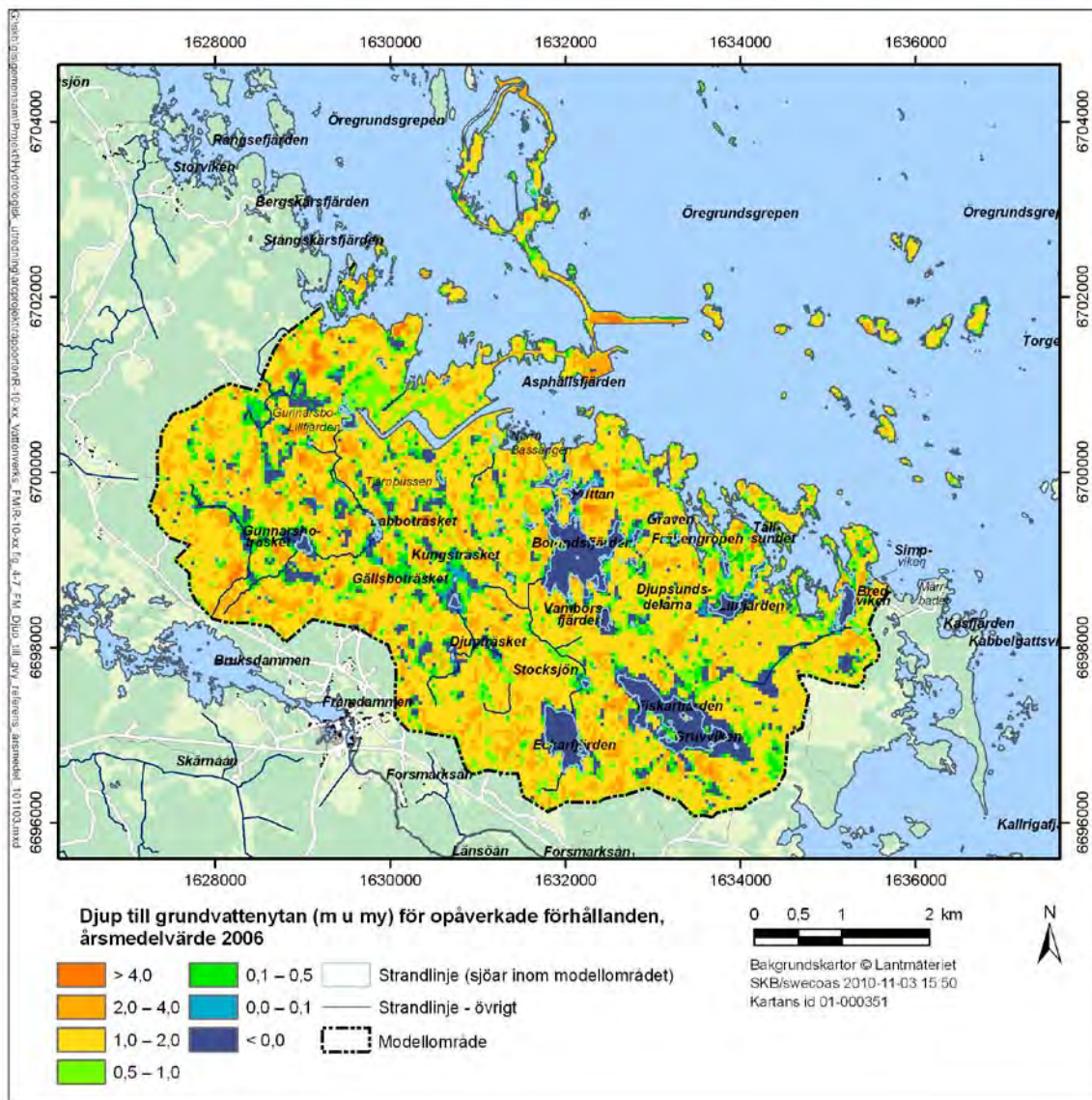
Figur 2-2. Årsmedelvärde på grundvattnens djup under markytan, beräknat med MIKE SHE-modellen för opåverkade förhållanden utan något förvar /Mårtensson och Gustafsson 2010/. Mörkblå områden (< 0,0) symboliserar ytvatten.
